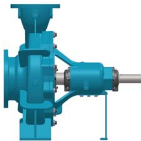
DS type - End Suction Heavy Duty
